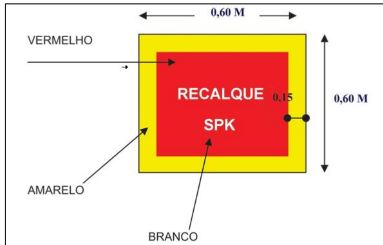
I – REGISTRO DE RECALQUE DE PAREDE
