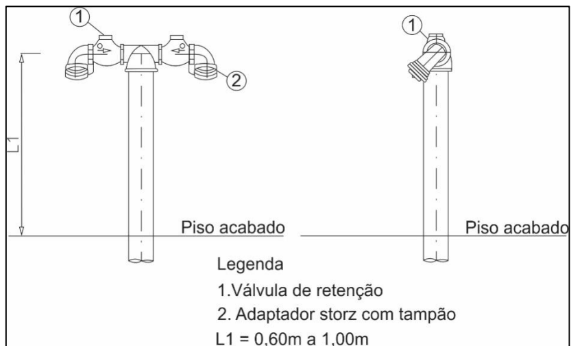
II – DISPOSITIVO DE RECALQUE TIPO COLUNA
